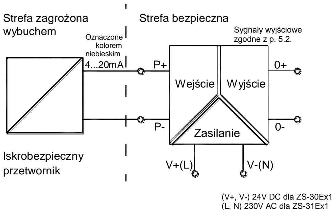
Rys.3. Schemat blokowy zasilacza-separatora ZS-30Ex1, ZS-31Ex1.
