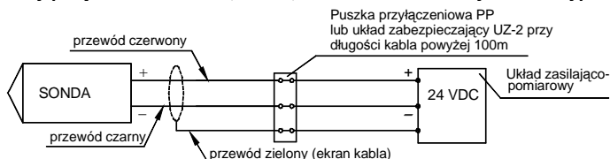
Rys. 3B. Schematy połączeń sond SG-25, SG-16, SG-25S i SG-25C w systemie dwuprzewodowym. (Nie dotyczy wykonania Ex)
