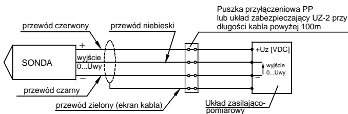
Rys. 3A. Schematy połączeń sond SG-25, SG-16, SG-25S i SG-25C w systemie trzyprzewodowym.
