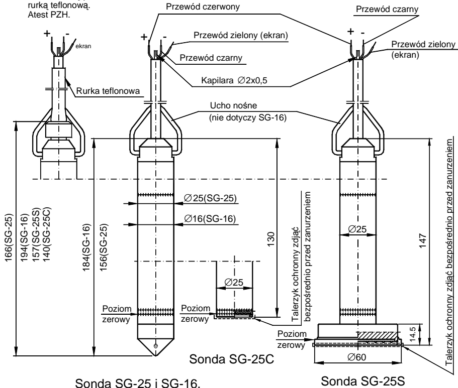
Rys. 3. Wymiary gabarytowe sond SG-25, SG-16, SG-25S i SG-25C.
