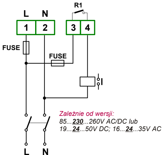
Rys. 4.9. Podłączenie zasilania oraz przełącznika sterującego obciążeniem
