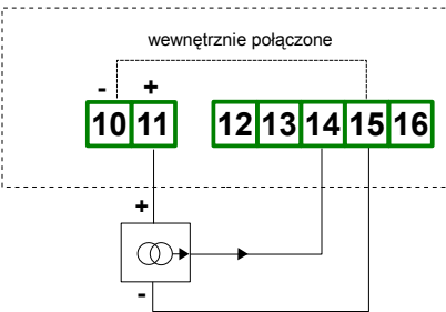
Rys. 4.7. Podłączenia przetworników prądowych 3 przewodowych
