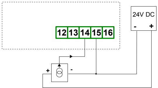
Rys. 4.7. Podłączenia przetworników prądowych 3 przewodowych
