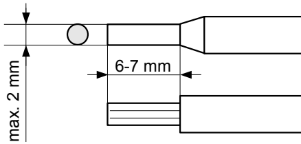
Rys. 4.3. Sposób odizolowania przewodów oraz wymiary końcówek kablowych
