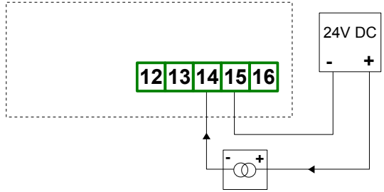
Rys. 4.6. Podłączenia przetworników prądowych 2 przewodowych
