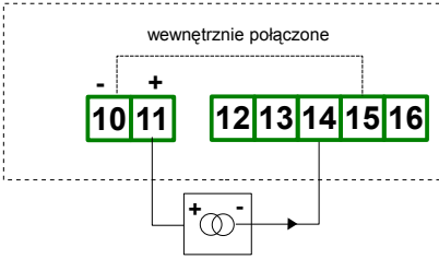
Rys. 4.6. Podłączenia przetworników prądowych 2 przewodowych
