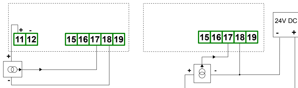
Rys. 4.9. Podłączenia przetworników prądowych 3 przewodowych
