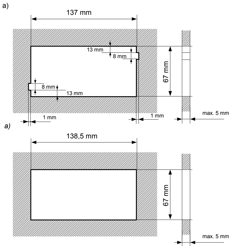
Rys. 4.1. Wymiary montażowe: a) zalecane, b) dopuszczalne
