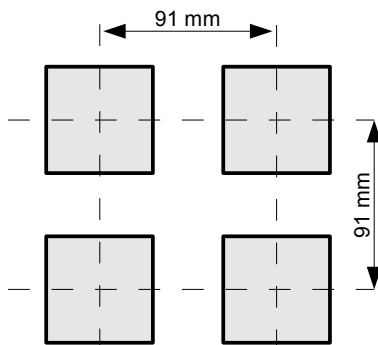
Rys. 4.2. Mocowanie za pomocą uchwytów
