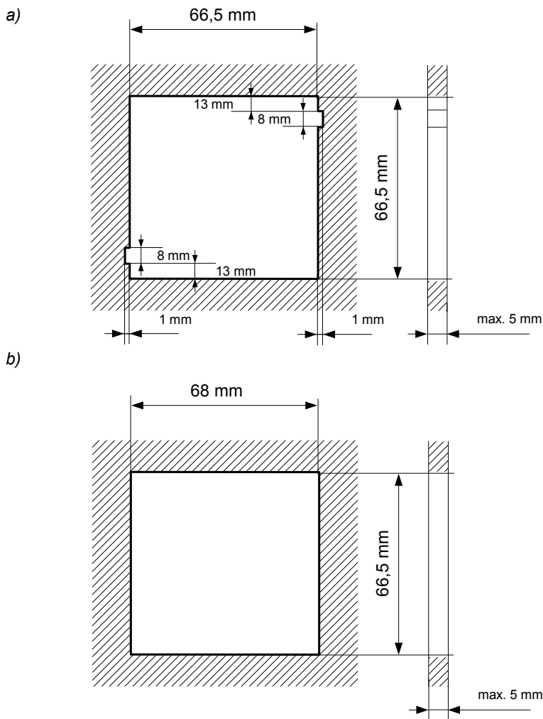
Rys. 4.1. Wymiary montażowe: a) zalecane, b) dopuszczalne
