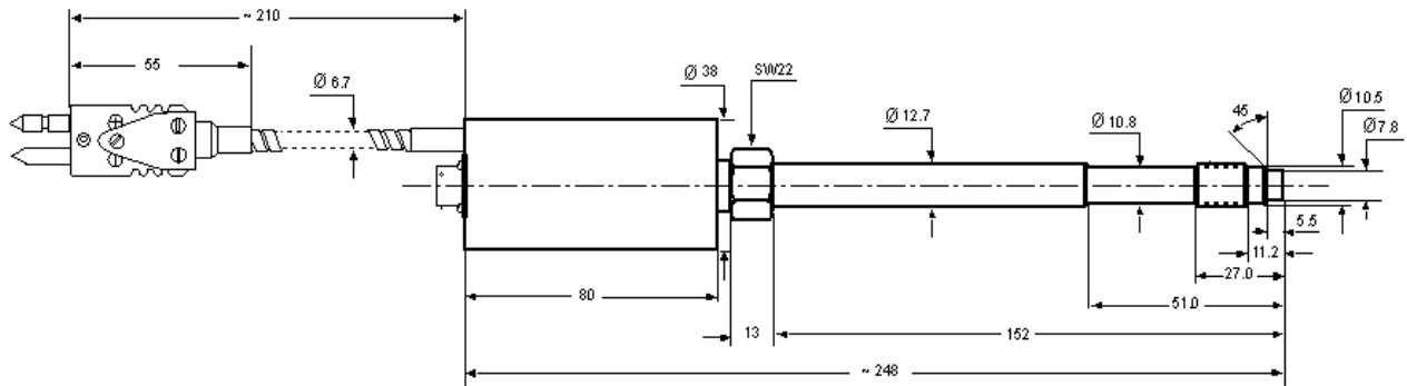
Wymiary przetwornika ciśnienia PC-38-CT
